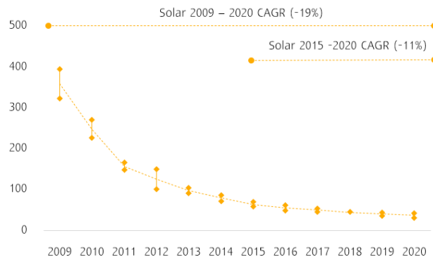
Levelized Cost of Energy (LCOE) ของ solar PV โดยไม่ให้ subsidy
