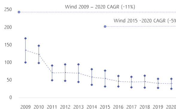
Levelized Cost of Energy (LCOE) ของพลังงานลมโดยไม่ให้ subsidy
